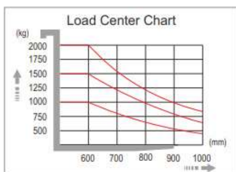
Рис.3 - График грузоподъемности CDDK10/CDDK12/CDDK15 Capacity (kg) – грузоподъемность (кг); Lift height (mm) – высота подъема (мм); load center (mm) – центр нагрузки (мм)
