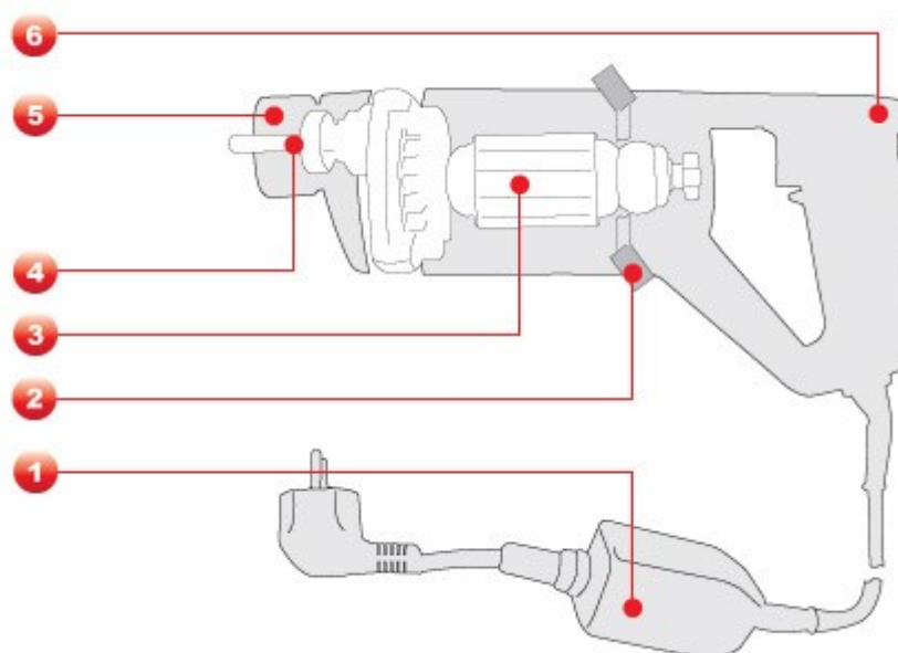
Рис.2 - Устройство электропривода
