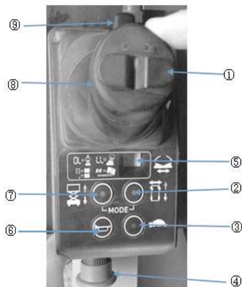
Рис. 2 - Контроллер платформы
