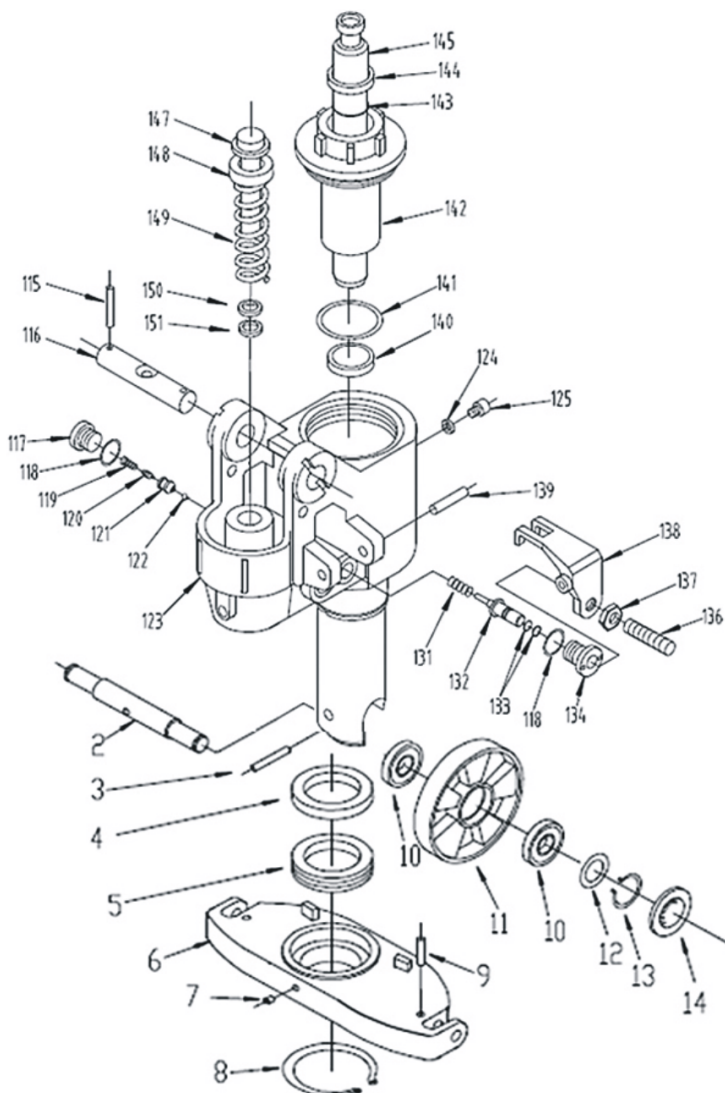
Рисунок 7. Гидравлический узел.
