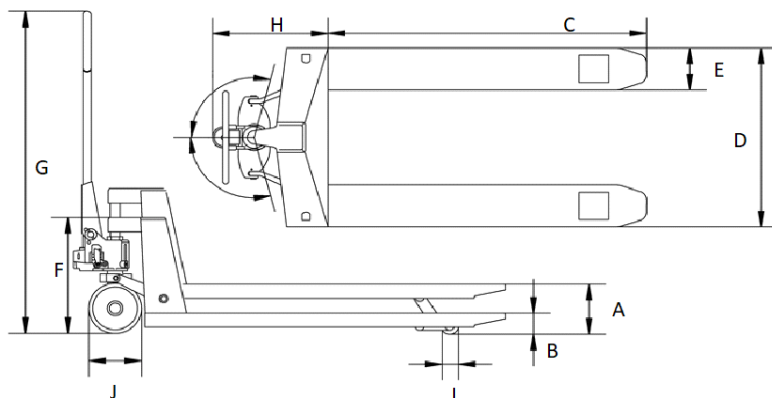
Рисунок 1. Размеры тележки.
