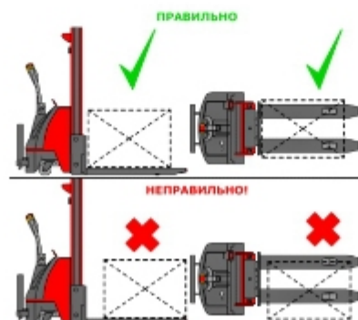
Рисунок 7. Схема расположения груза на вилках.
