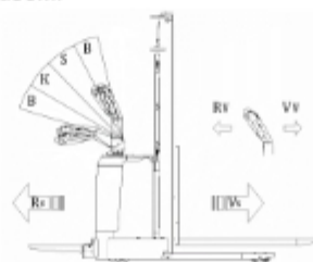
Рисунок 6. Положение румпеля управления.
