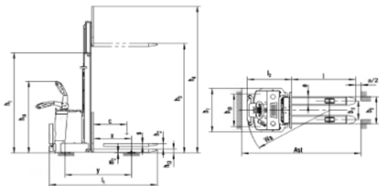
Рисунок. 4 Основные параметры штабелера.
