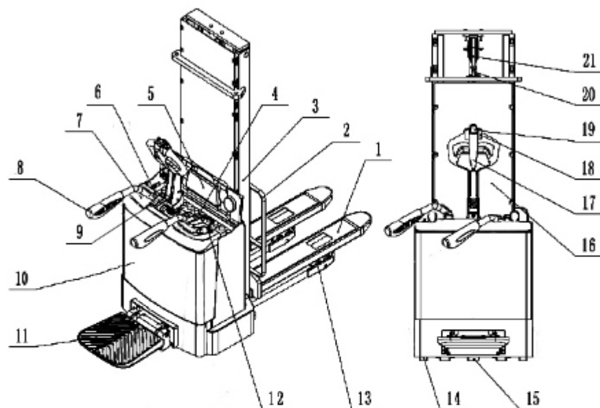
Рисунок 1. Обзор основных компонентов.
