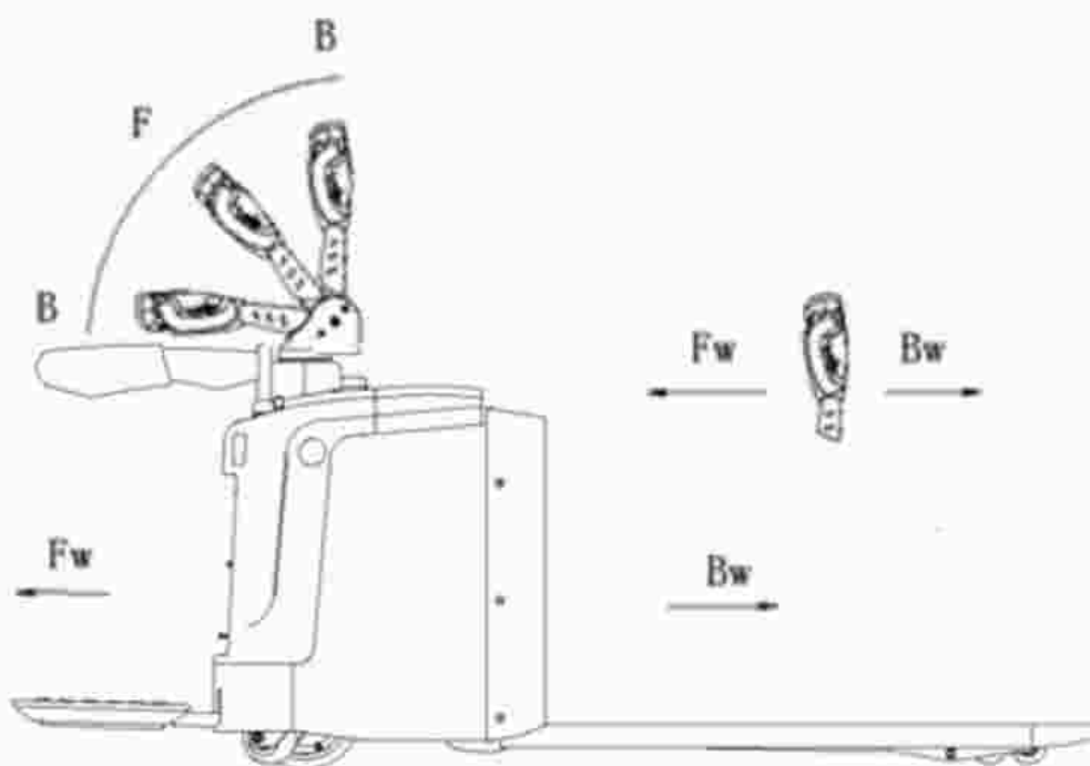
Рисунок 4. Управление тележкой.
