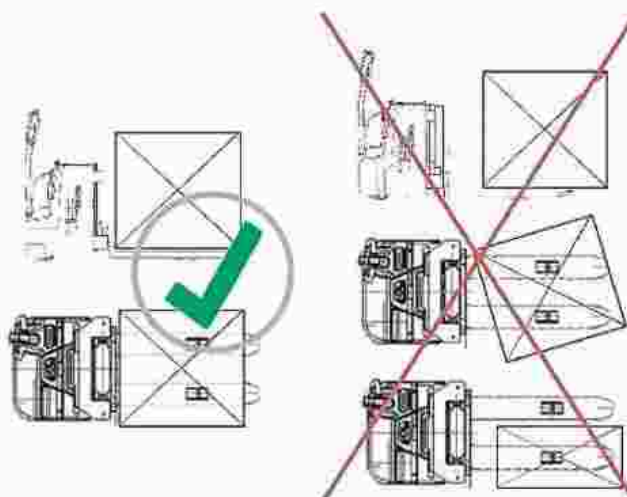
Рисунок 5. Схема расположения груза на вилах
