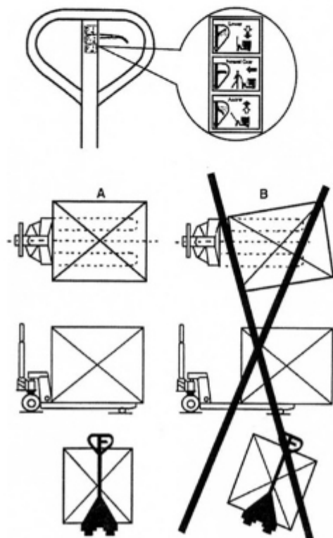
Рисунок 7. Расположение груза.
