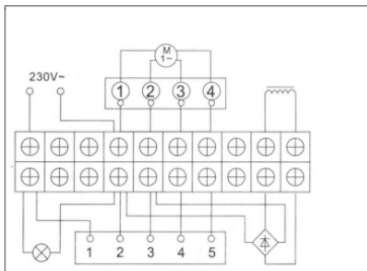
Рисунок 3. Электрическая схема пульта управления
