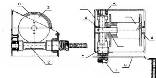
Рисунок 3. Спецификация лебедки модели HWG.
