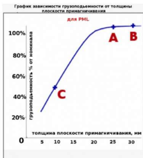
Рисунок 4. Факторы, влияющие на грузоподъемность магнитных захватов.
